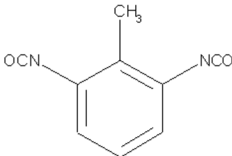
2,6-TDI
